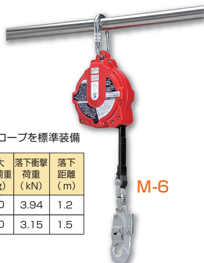
安全ブロック 6m
