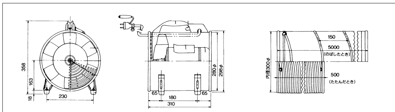
標準形送風機の構造と外形寸法 PF-281
